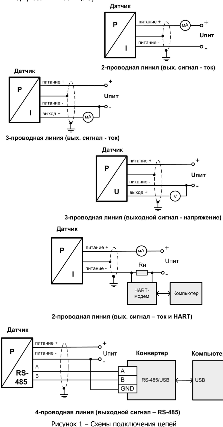
Рисунок 1 – Схемы подключения цепей
