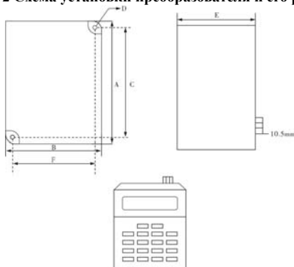
3-2 Схема установки преобразователя и его размеры
